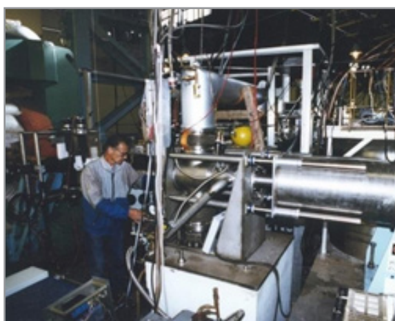
Figure 9: Movable polarized target, N. S. Borisov, 1995 LHE, JINR
